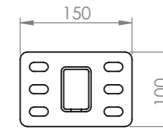
M10 Bolzenanker
